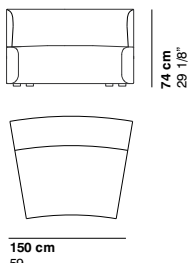
COD.1469 ELEMENT 150
