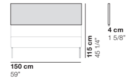
cod. 1213 / back panel 150 h. 115
