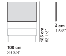
cod. 1212 / back panel 100 h. 135
