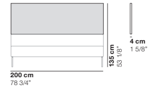
cod. 1216 / back panel 200 h. 135
