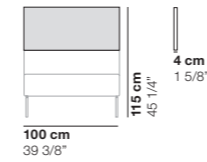
cod. 1211 / back panel 100 h. 115
